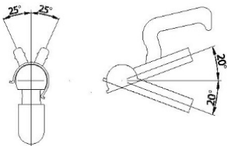
Bild 3: Schwenkbereich
