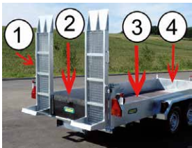
Bild: Baumaschinen Anhänger hinten
